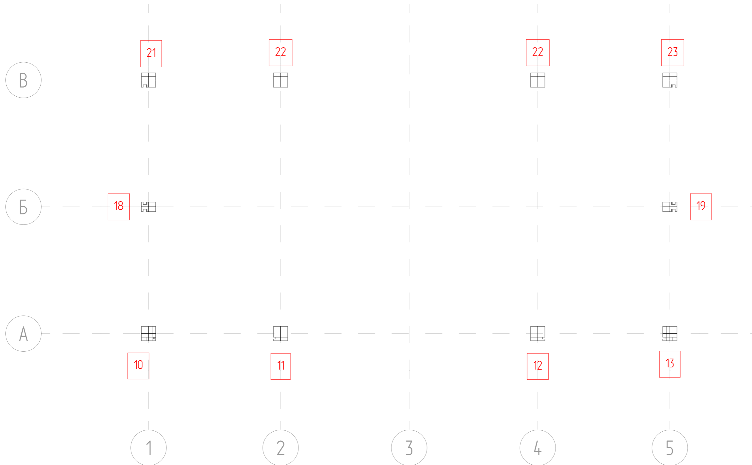
Спецификация - Стойки
